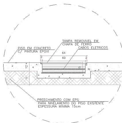
DETALHE CANALETA PISO
